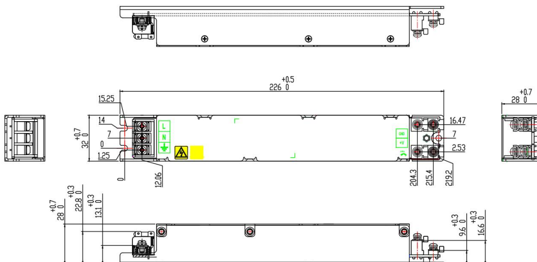
外形尺寸及安装孔——端子坐标
